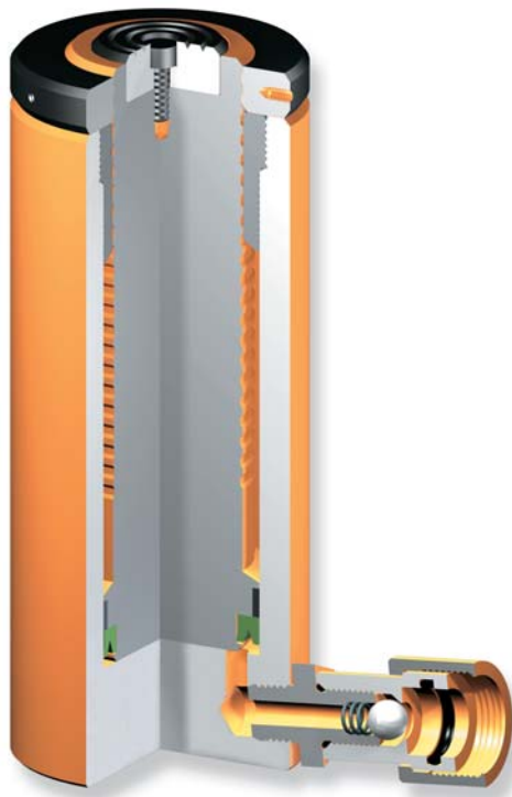
Detalle de construcción
