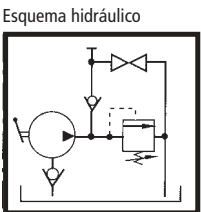
Esquema hidráulico
