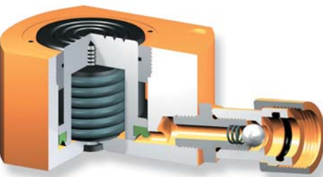
Detalle de construcción
