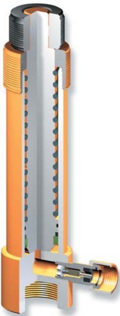
Detalle de construcción (CC)
