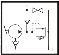
Esquema hidráulico
