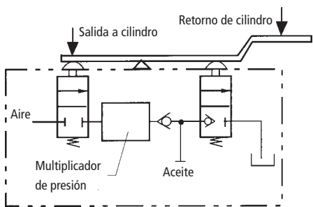
Esquema de funcionamiento
