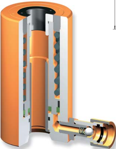
Detalle de construcción (CSH)
