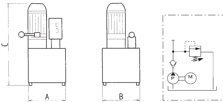
Esquema hidráulico
