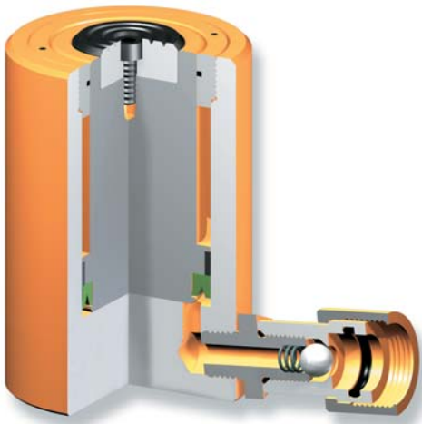
Detalle de construcción
