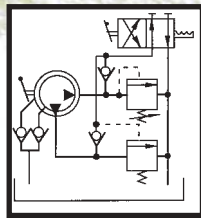
Esquema hidráulico
