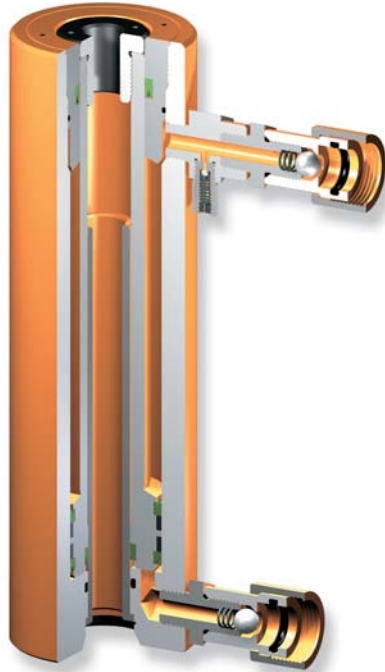
Detalle de construcción (CDH)
