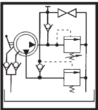
Esquema hidráulico
