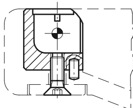
Ejemplo de montaje normal con base saliente
