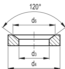
DIN 6319-D (d4=d2) (arandela cóncava)
